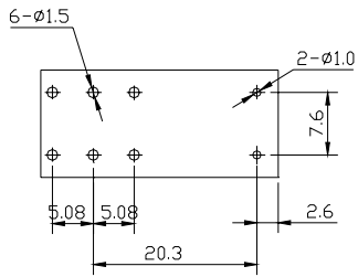
安装图
