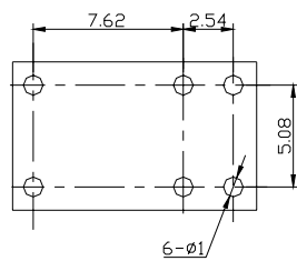
安装图
