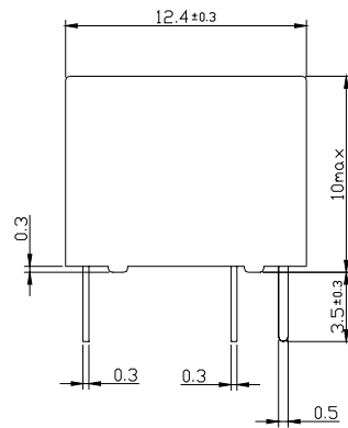
安装图
